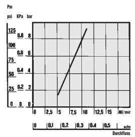
MINIMUM DURCHFLUSS-DIAGRAMM
